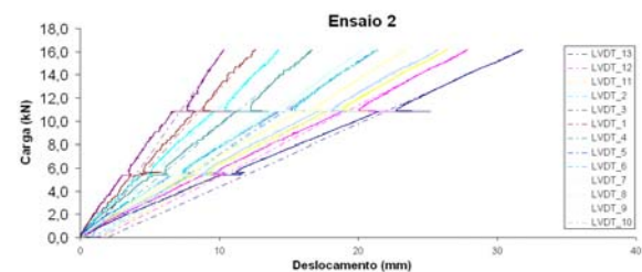
Fig. 11 – Gráfico carga-deslocamento para as 5 vigas do ensaio de carga 2.
