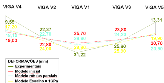
Fig. 15 – Comparação das deformações a meio vão das vigas obtidas no ensaio E1 para as várias modelações numéricas.
